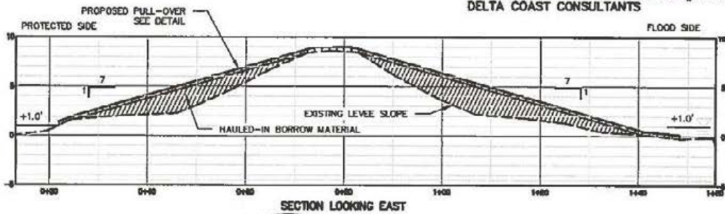
EAST PIROQUE PULL-OVER - SECTION B-B (N.T.S.)
