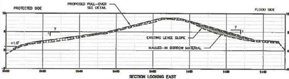
WEST PIROQUE PULL-OVER - SECTION C-C (N.T.S.)
